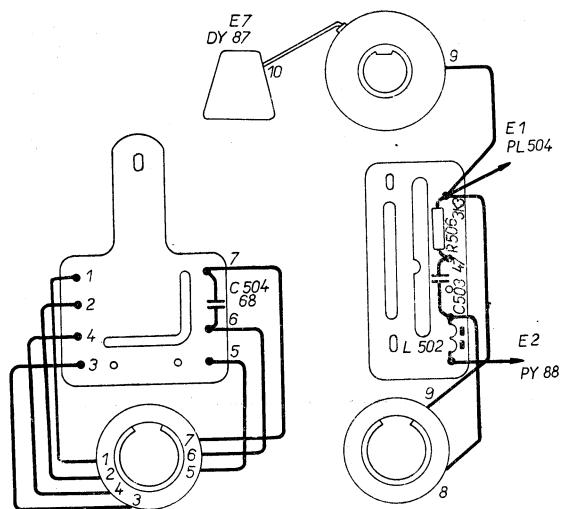
Obr. 13. Vysokonapäťové trafo 6PN 3 0 20
