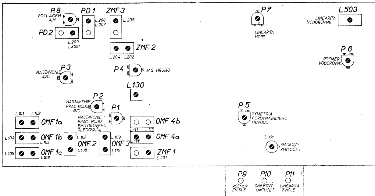
Obr. 6. Rozmiestnenie ovládacích prvkov a doladovacích jadier
