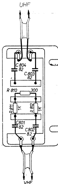
Obr. 14. Anténne zdiery 6PF 683 67
