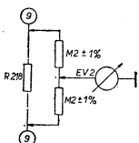
Obr. 8b. Pripojenie EV pri ladení PD
