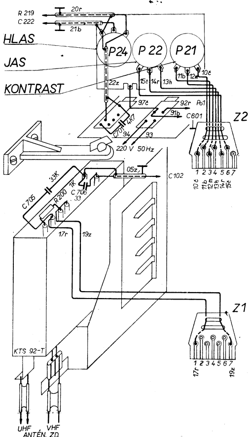
Obr. 10. Zapojenie bočnika SPOLETO
