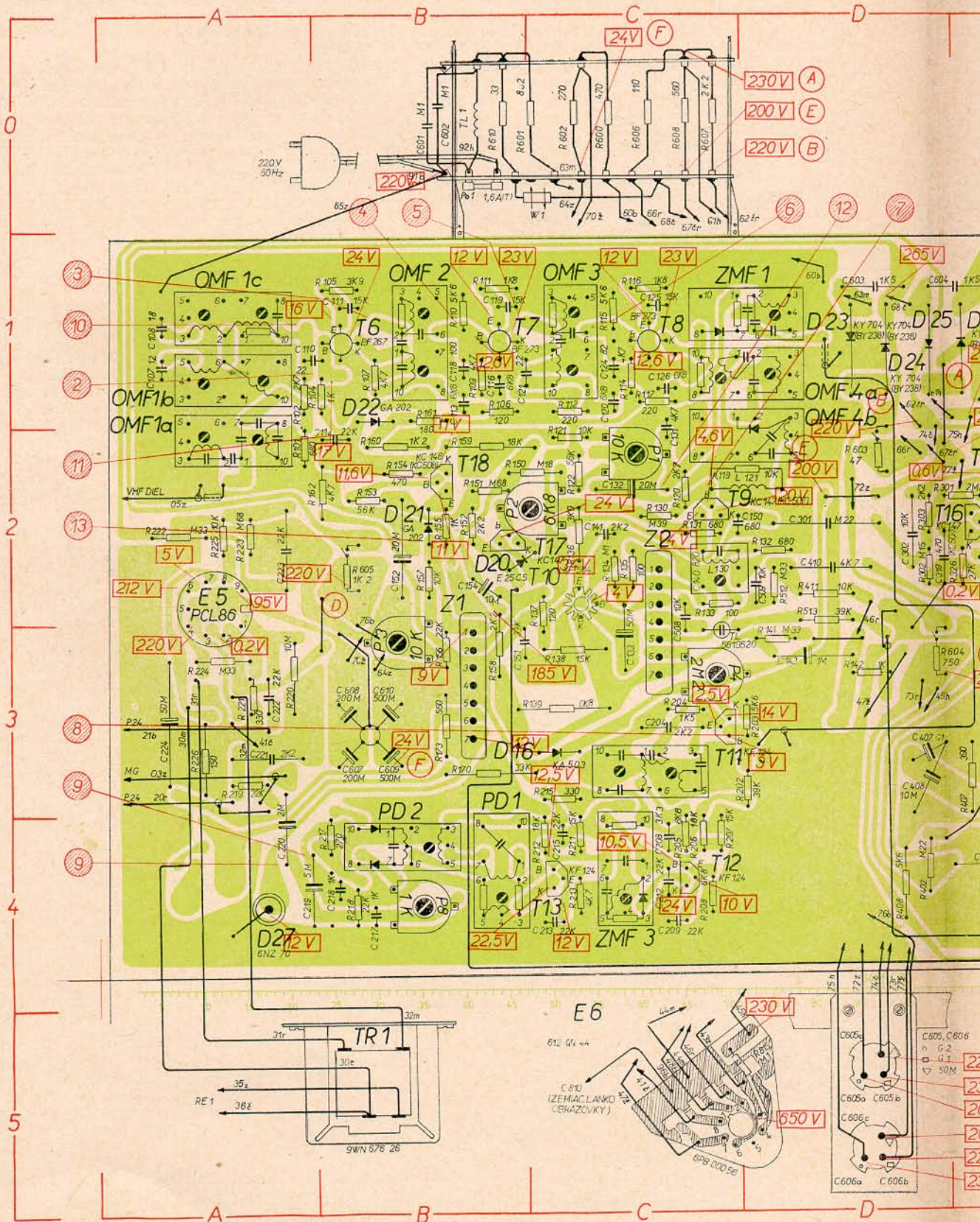
Obr. 24. Chassis zostave
