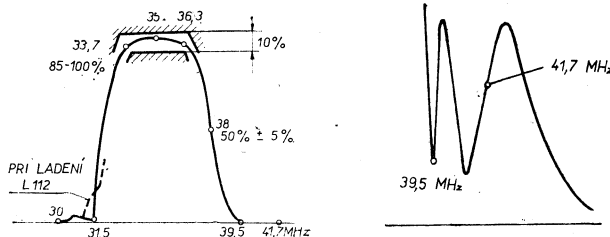
Obr. 7. Celková krivka OMF a jej detail
