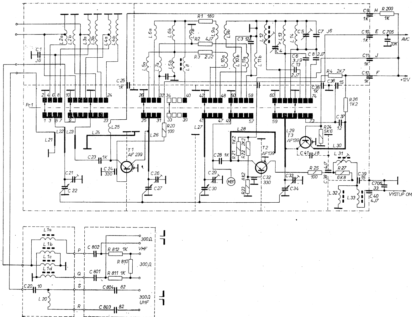
Obr. 21. Elektrické zapojenie kanálového voliča
