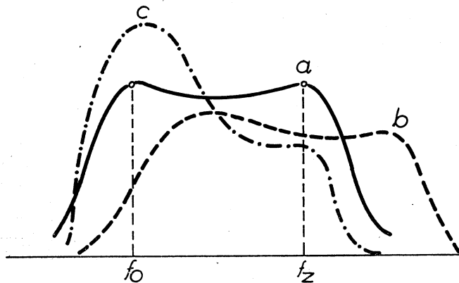
Obr. 18. Kontrola priebehu charakteristiky na pásmach UHF
