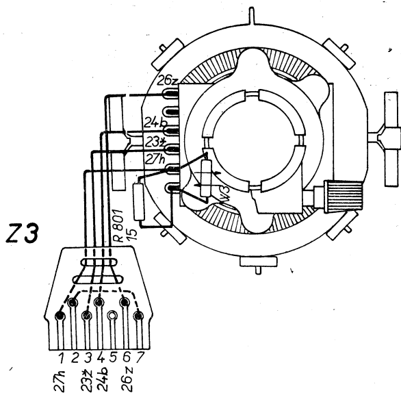
Obr. 12. Vychyľovacia jednotka 6PN 0 0 95
