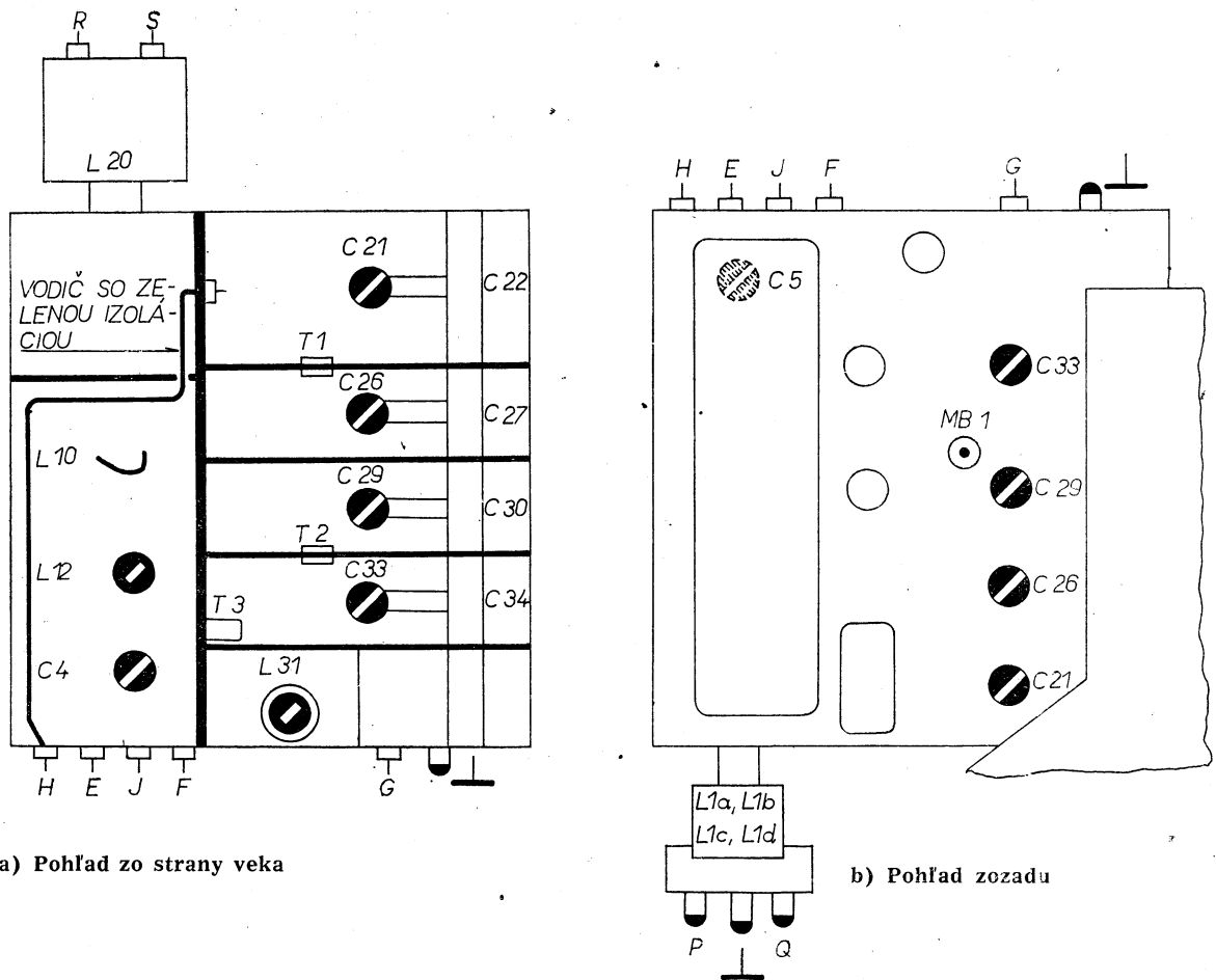
Obr. 20. Nastavovacie prvky kanálového voliča
