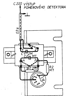
Obr. 15. Magnetofónová prípojka 6PN 051 15
