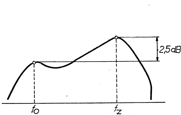
Obr. 19. Prípustná tolerancia tvaru krivky
