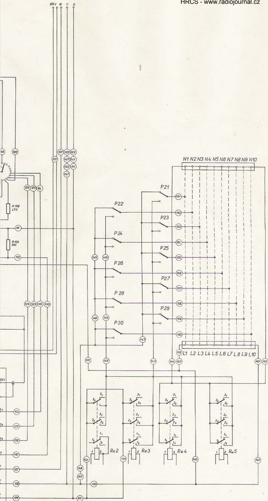
RELE RE 1 ÷ 5 TYP RP 402
