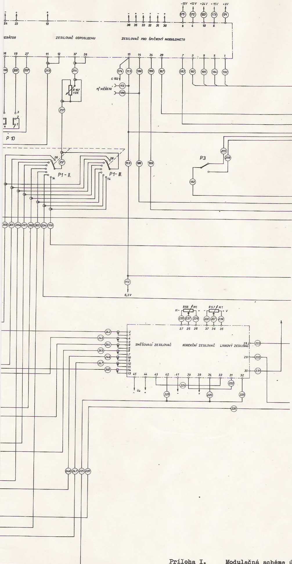
Príloha I. Modulačná schéma ústredne
