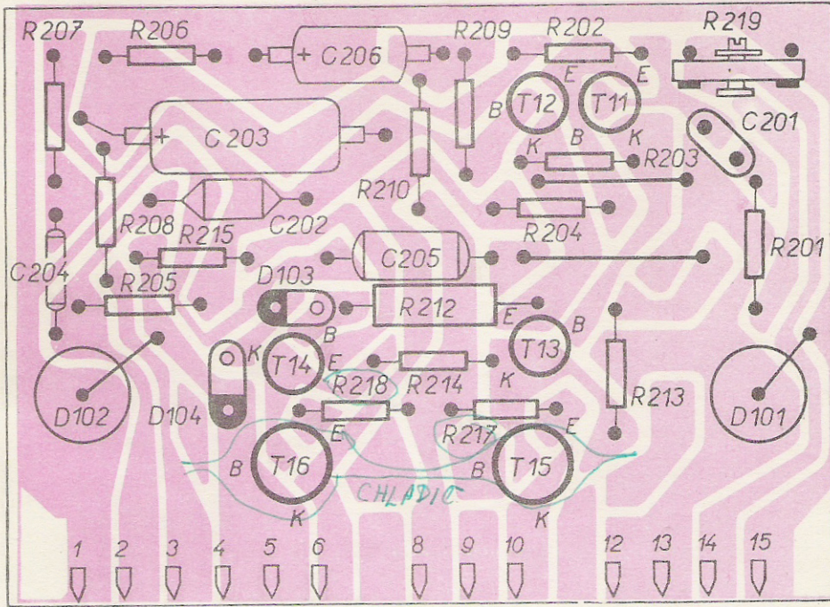
Priloha X. Doska vstupného zosilňovača
