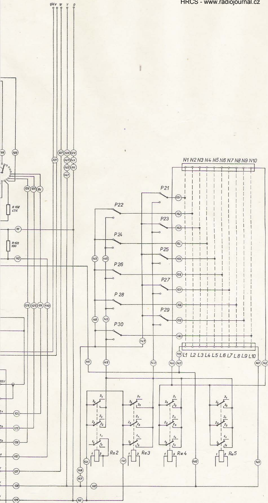
RELÉ RE 1 ÷ 5 TYP RP 102
