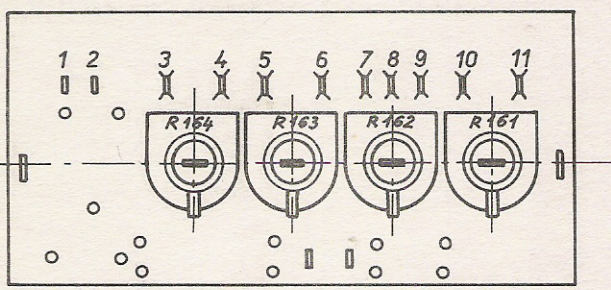
Príloha IV. Doska s potenciometrami
