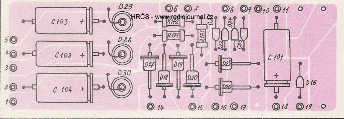
Príloha III. Napájacia doska 3AK 060 74
