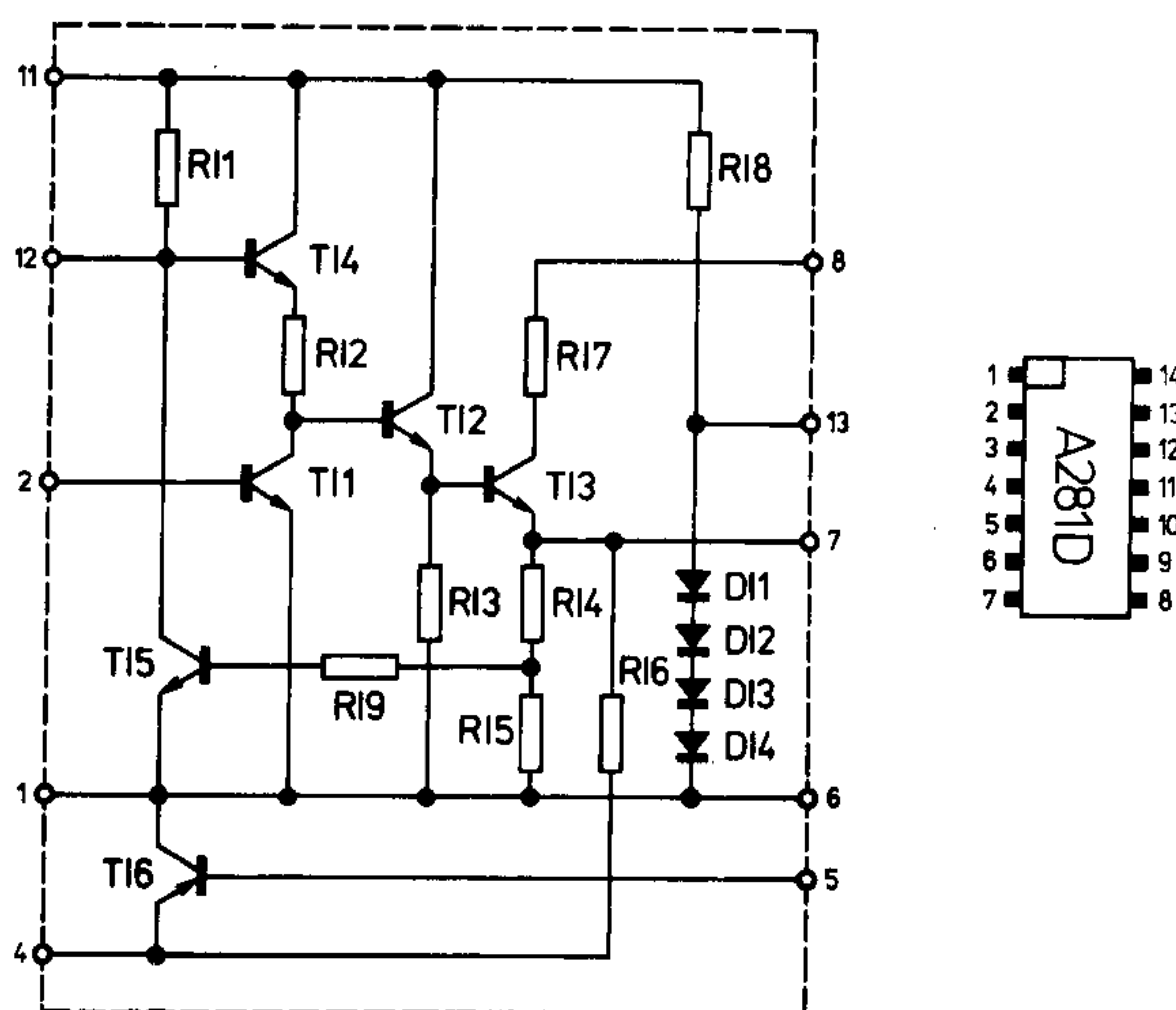
Obr. 2. Zapojení integrovaného obvodu IO3
